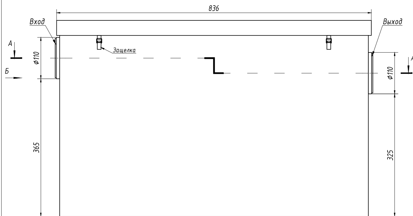
Вид спереди
