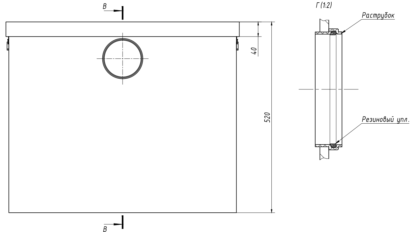
Вид Б
